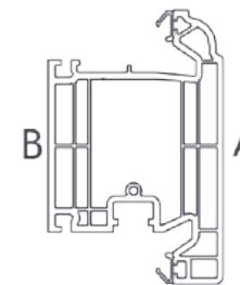
705541 Door Sash Open Out
