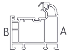
705809 68mm Composite Door Outerframe
