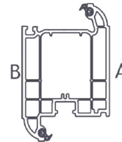
105168 110mm Z Door Sash
