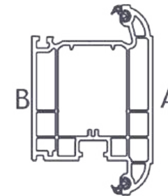
105169 110mm T Door Sash
